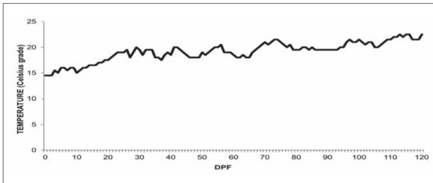
1. ábra. A „hideg kamra” vízhőmérsékleti görbéje. Figure 1. Water temperatures in the „cold room”.
