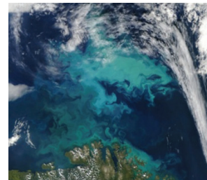
Fitoplankton túlszaporodása a Barrents tengeren Norvégia mellett
